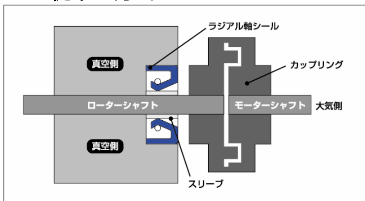
標準的なドライブ機構
