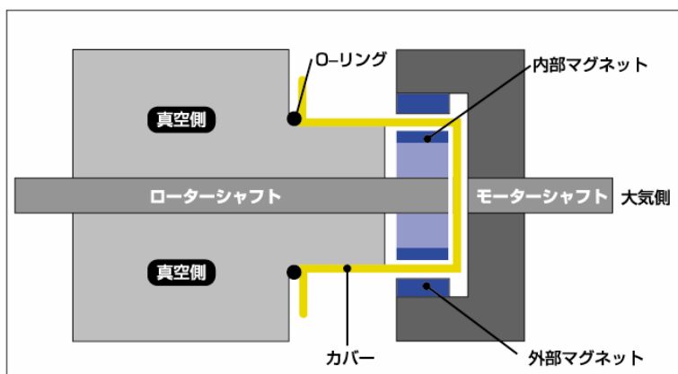
シール材が消耗しない新機構、マグネットカップリング
